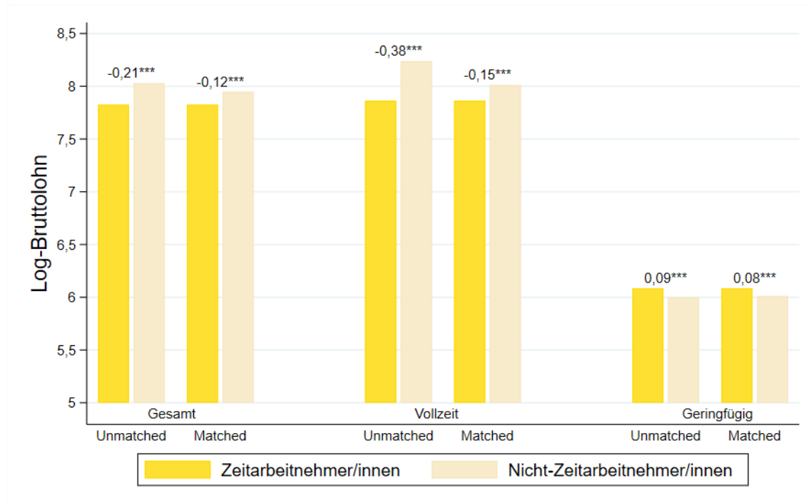
ABBILDUNG 11: STATISTISCHE ZWILLINGE AUF DER GRUNDLAGE VON PROPENSITY SCORE MATCHING, MODELL 5, MONATSLOHN
